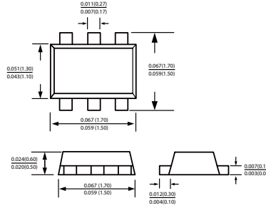
SOT-563
