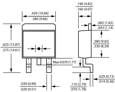
D2-PAK
