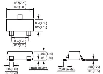
SOT-323
