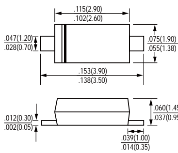
SMF
