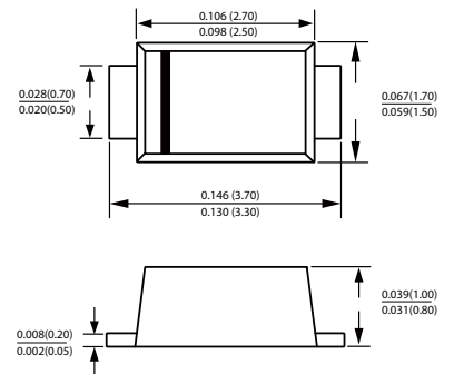
SOD-123L
